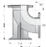
N Flanschfußbögen
