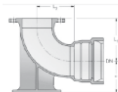
EN Hydrantenfußbögen
