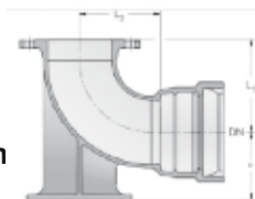
EN Hydrantenfußbogen
